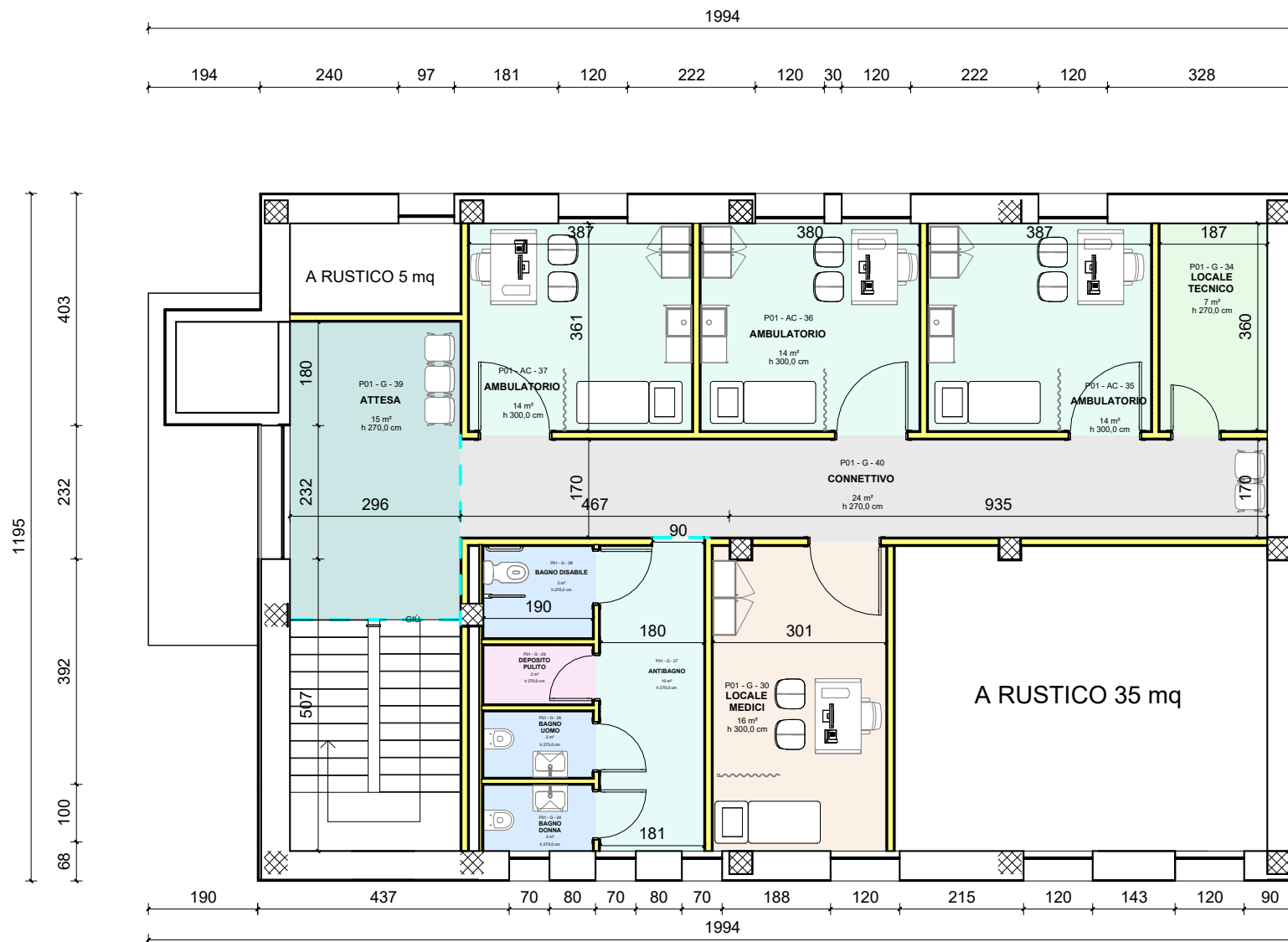
DISTRIBUZIONE FUNZIONALE PIANO PRIMO SCALA 1:100
